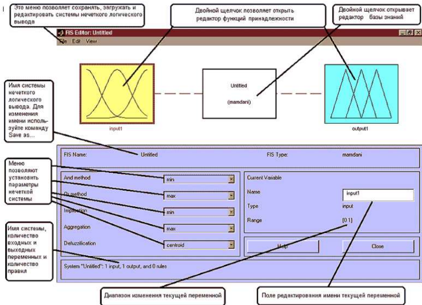
Рис. 2. Окно редактора FIS-Editor
