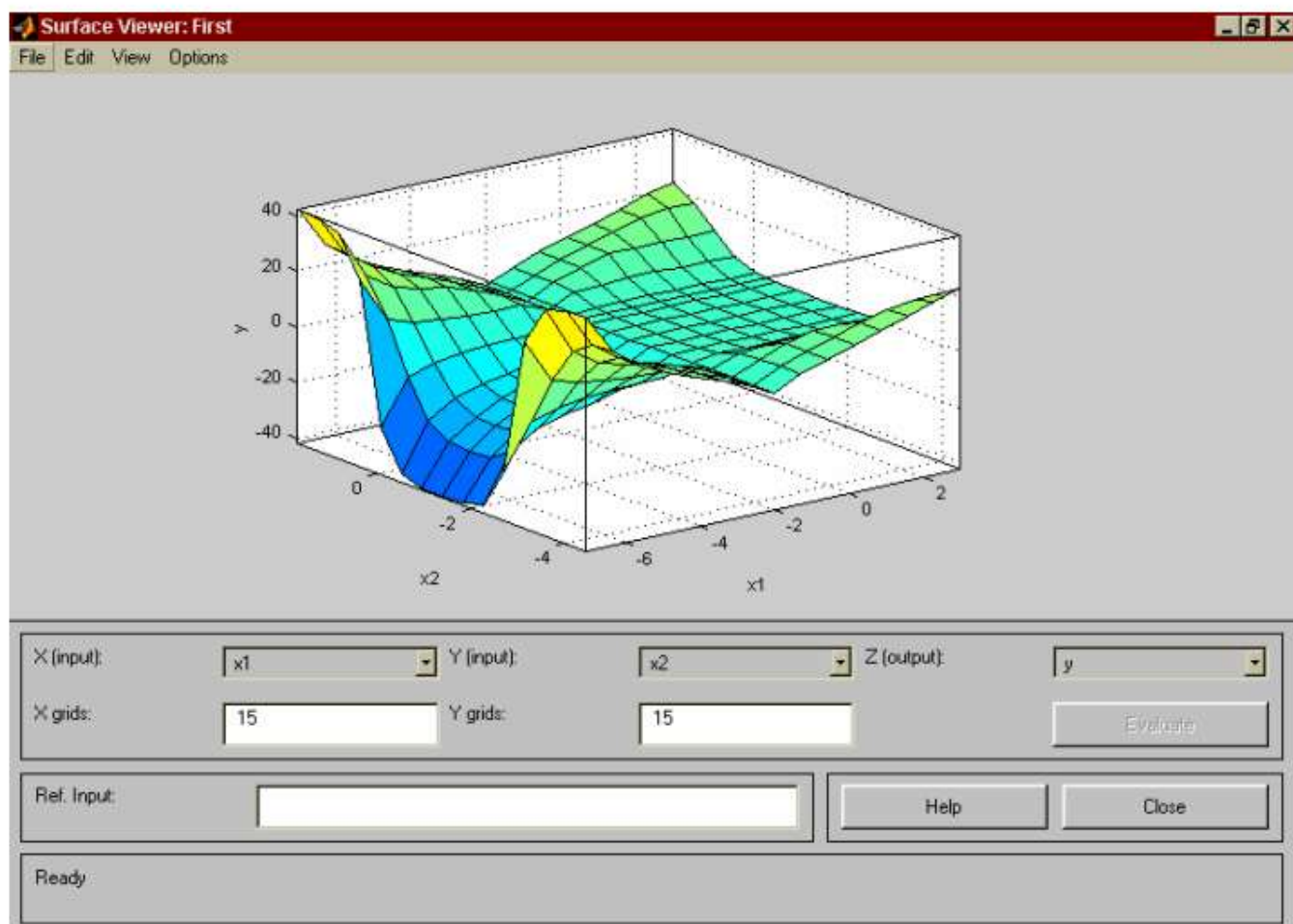
Рис. 8. Поверхность “входы-выход” в окне SurfaceViwer
